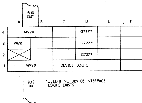
DD11-A Module Layout
